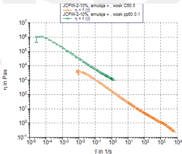
Rys. 4. Porównanie krzywych lepkości emulsji, zawierającej układ wosków Jeepsperse CPW-2 oraz Natural WaxJelly
