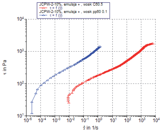
Rys. 3. Porównanie krzywych płynięcia emulsji, zawierającej układ wosków Jeepsperse CPW-2 oraz Natural Wax Jelly
