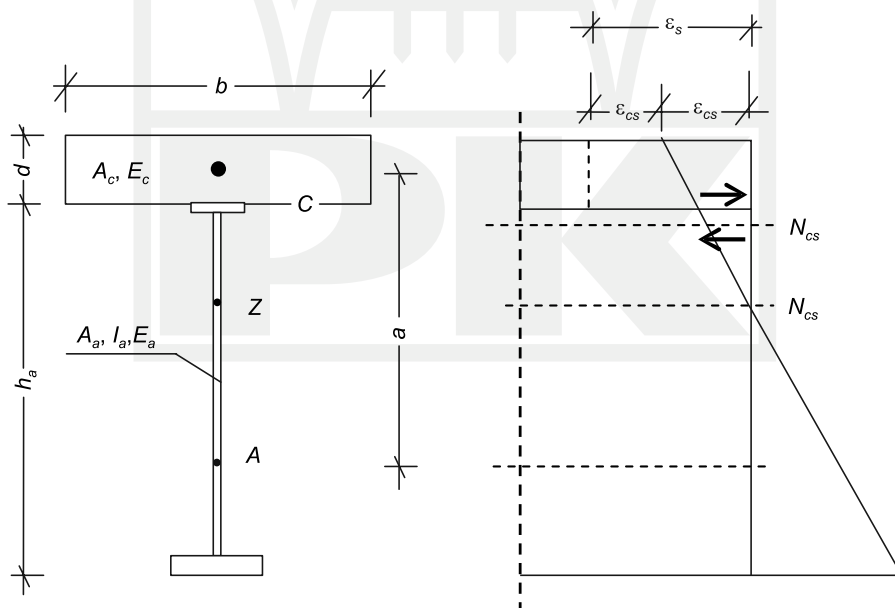
Rys. 3. Odształcenia skurczowe dla przypadku ogólnego
