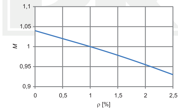
Rys. 6. Wpływ procentu zbrojenia płyty \rho na wartość współczynnika M
