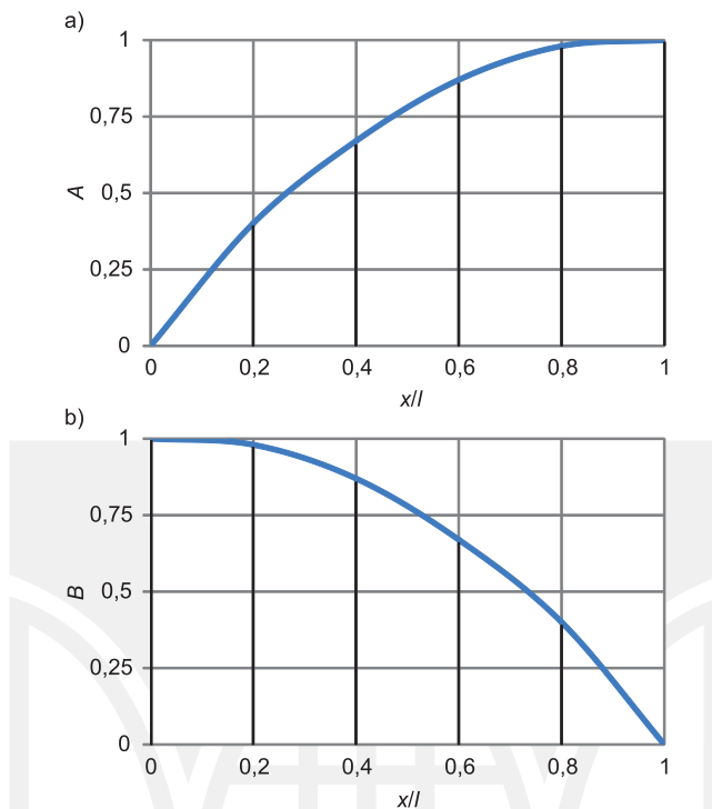
Rys. 5. Przebieg zmian wartości naprężeń na długości elementu: a – naprężenia normalne, b – naprężenia styczne
