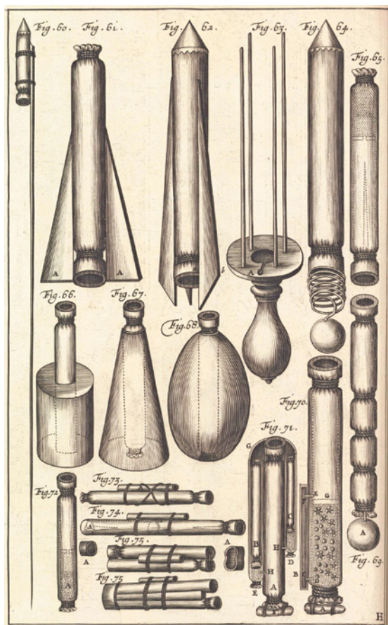
II. 3. Karta przedstawiająca projekty rakiet z dzieła Artis magnaë artilleriæ pars prima Kazimierza Siemienowicza, 1650
